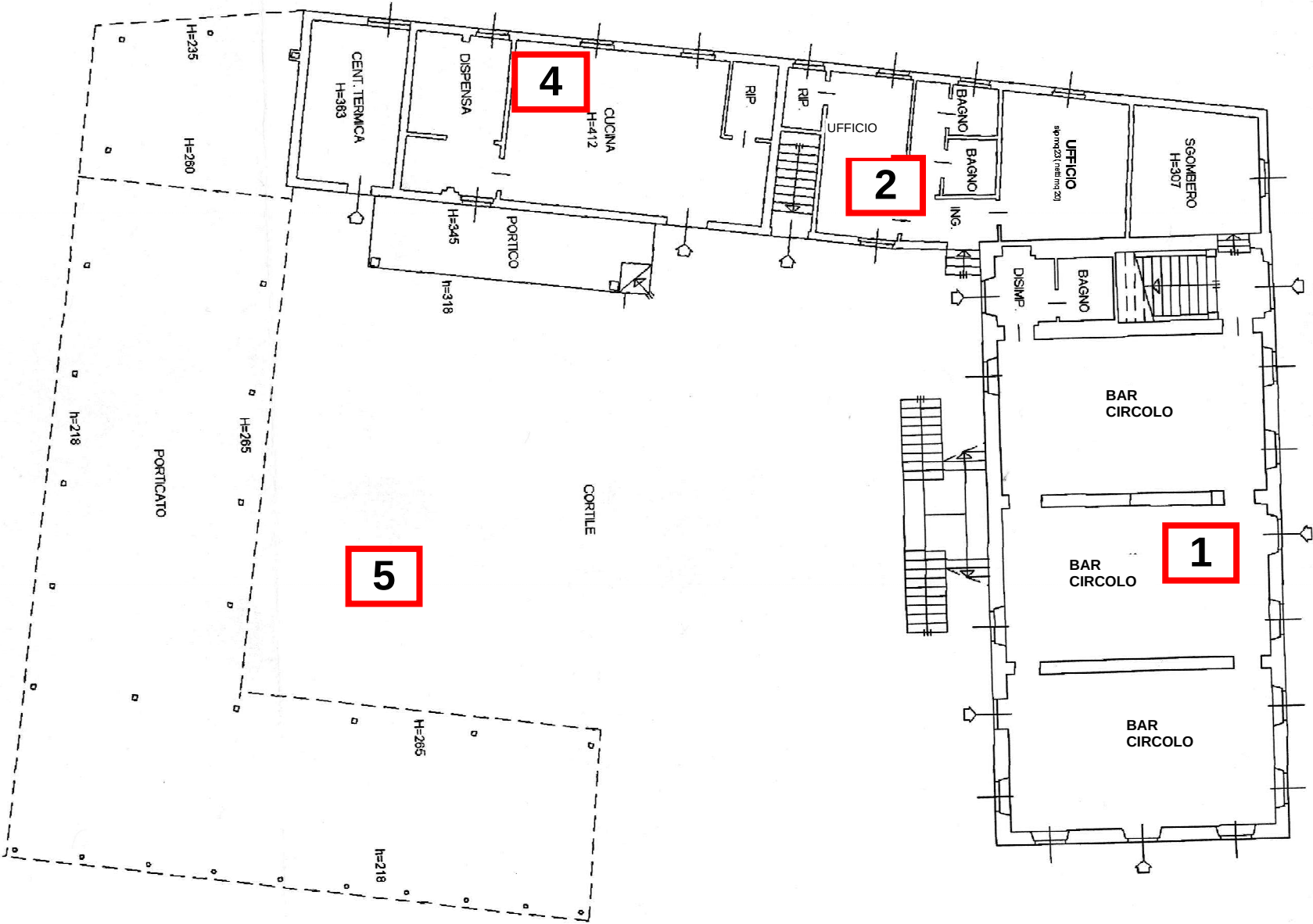
Planimetria 1: 200
